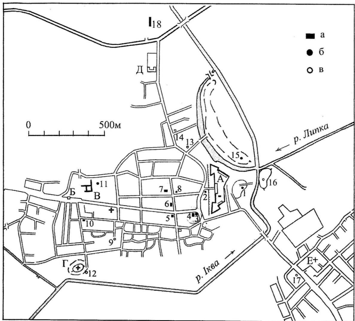
Рис. 1. План центральної частини м. Дубна.
